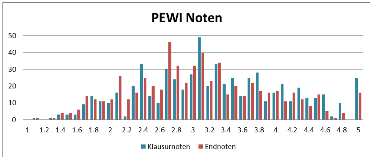
Abbildung 1: Verteilung der Klausurnoten, absolute Häufigkeiten
